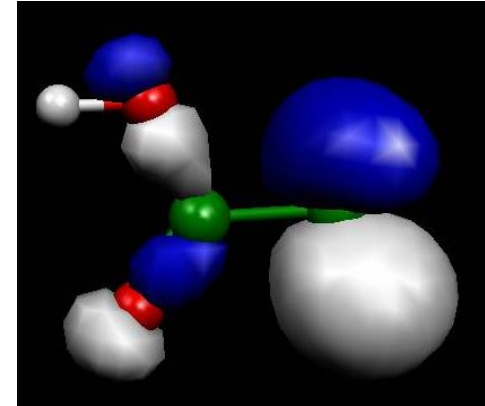
Orbitais moleculares
