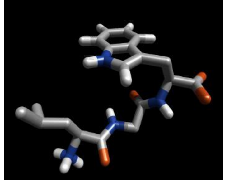
Tripéptido Leu-Gly-Trp
