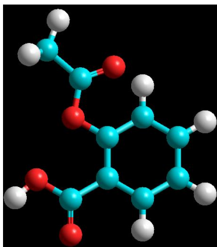
Coordenadas atómicas
