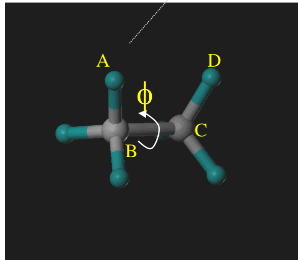
Etano
