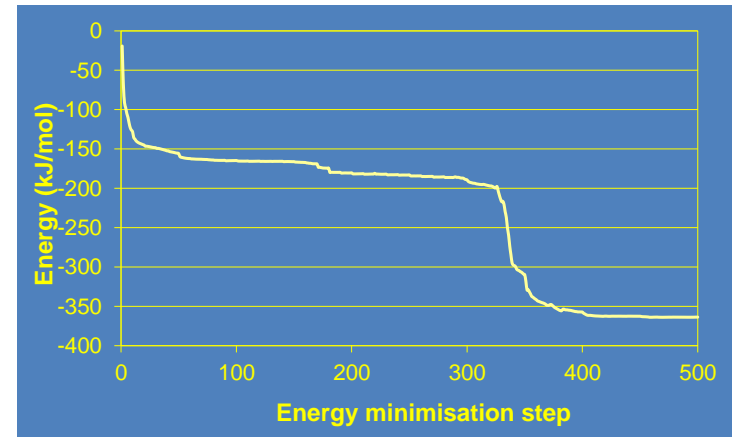
Tripéptido Leu-Gly-Trp
