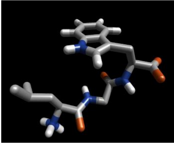
Conformação inicial
